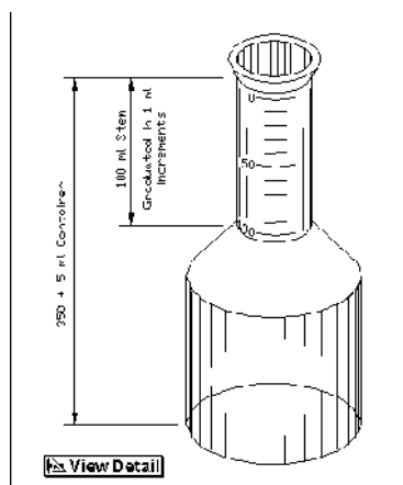
Pycnometer FIG. 4
